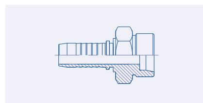
Male Metric French Serie 24° Cone Seat (AGF) 23.1200
