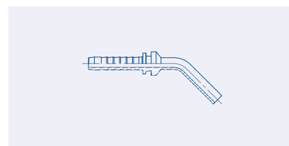
45° Swept Metric Standpipe (BEL 45) 23.6040
